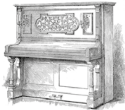
Modèle 6. PIANO DROIT à 7 octaves \frac{1}{2} de la à l'a à Cordes croisées — Châssis en métal — Sonnetier recouvert de métal — Mécanique à répétition. Hauteur 1 m 50 — Largeur 1 m 45 — Profondeur 0 m 69
